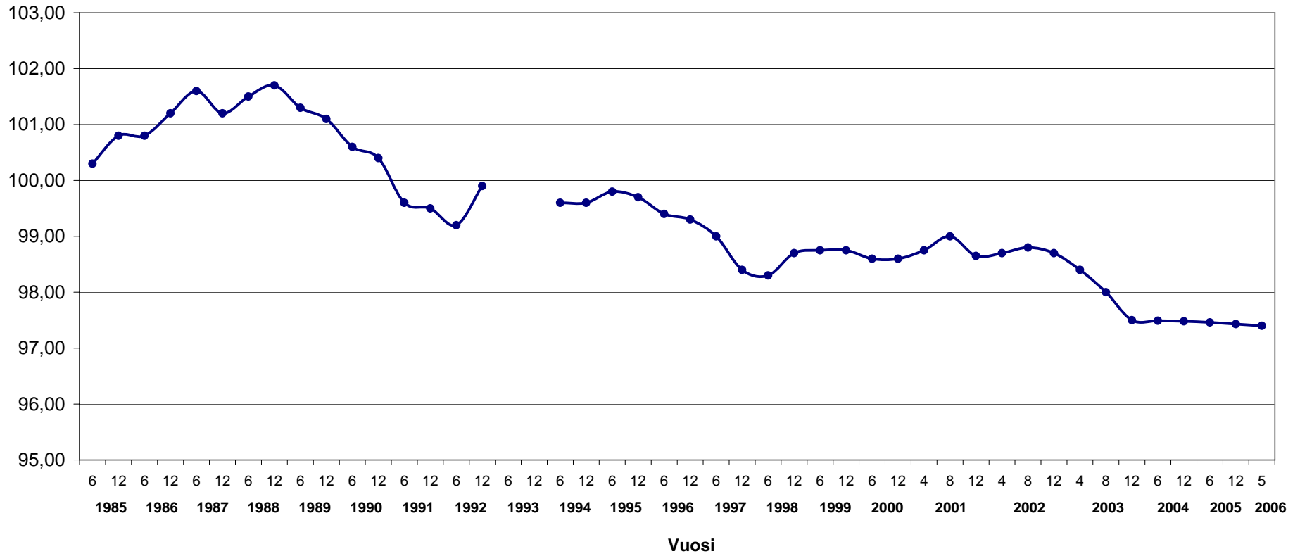
Kinnalan vedenottamon vedenpinnan korkeus vuosina 1985-2006
